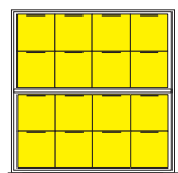
16 plastic bins 6" w x 6" d & partition NFCC0453030 04 & 05 NFCC0673030 06 & 07
